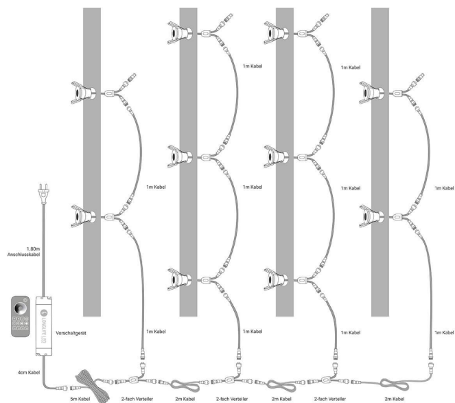
Einbaustrahler 10er Set Installationsbeispiel 3
