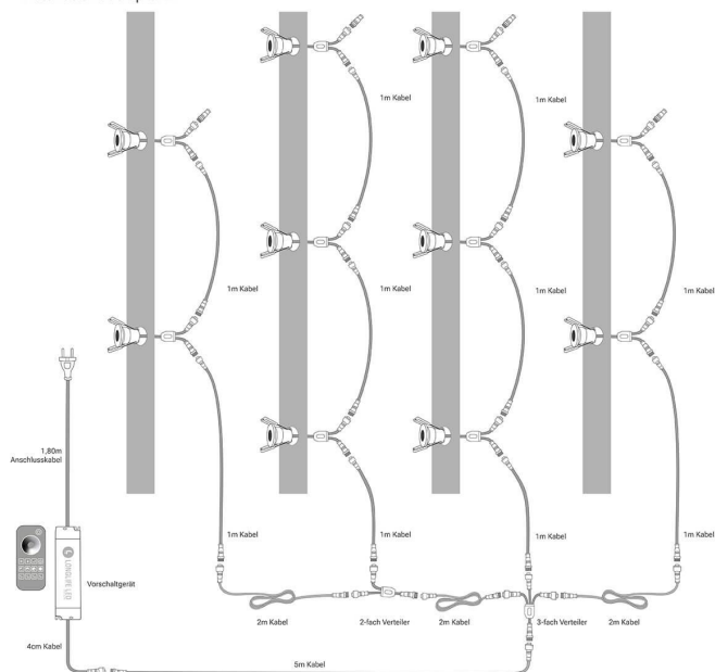
Einbaustrahler 10er Set Installationsbeispiel 2
