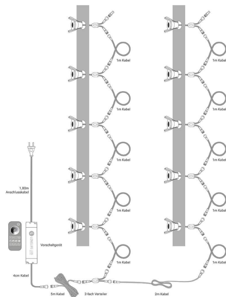
Einbaustrahler 10er Set Installationsbeispiel 1
