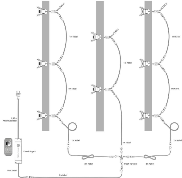
Einbaustrahler 8er Set Installationsbeispiel 1
