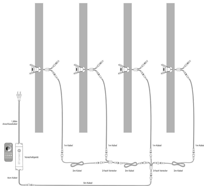
Einbaustrahler 4er Set Installationsbeispiel 2
