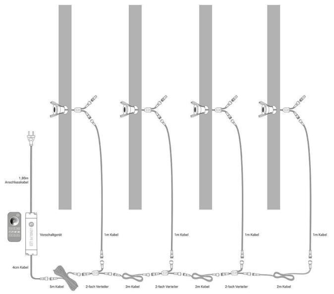
Einbaustrahler 4er Set Installationsbeispiel 3
