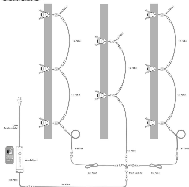
Einbaustrahler 8er Set Installationsbeispiel 1
