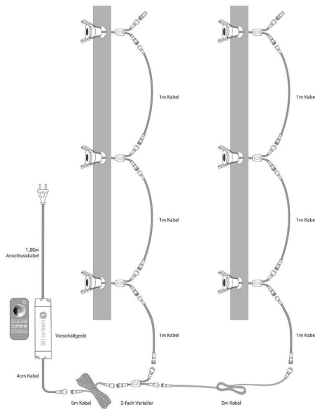
Einbaustrahler 6er Set Installationsbeispiel 3
