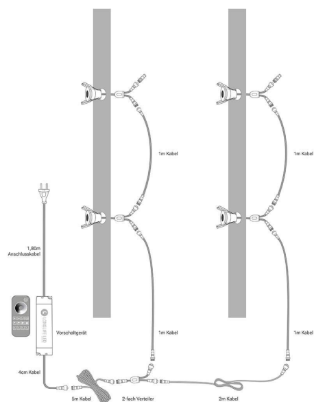
Einbaustrahler 4er Set Installationsbeispiel 1
