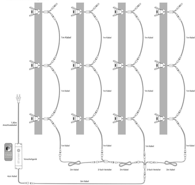
Einbaustrahler 12er Set Installationsbeispiel 2
