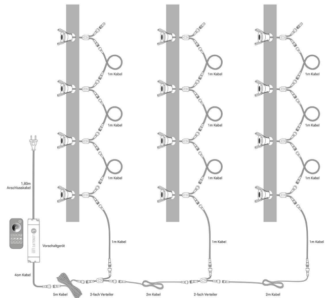
Einbaustrahler 12er Set Installationsbeispiel 3
