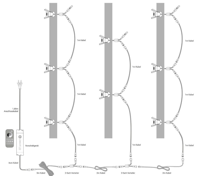
Einbaustrahler 8er Set Installationsbeispiel 2
