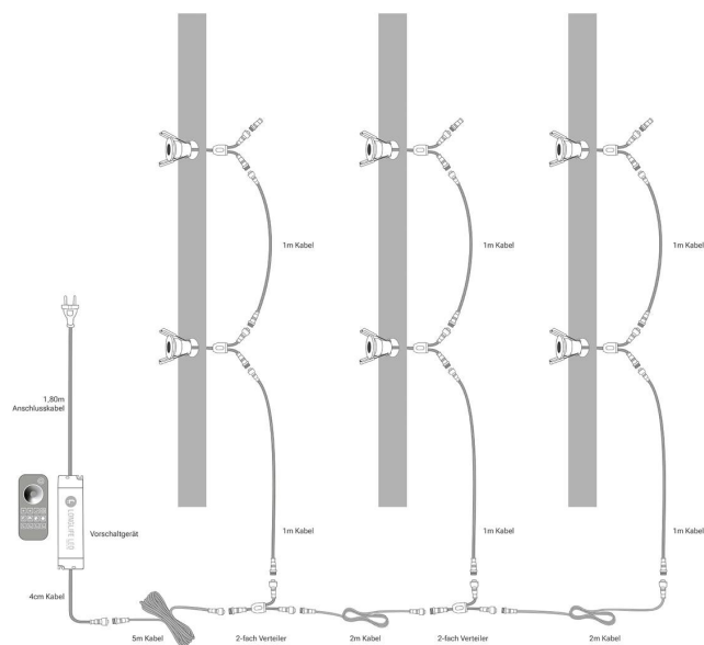
Einbaustrahler 6er Set Installationsbeispiel 2
