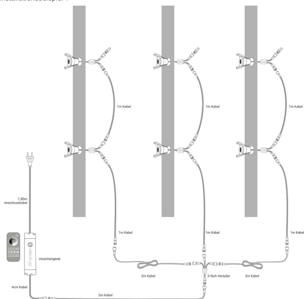
Einbaustrahler 6er Set Installationsbeispiel 1
