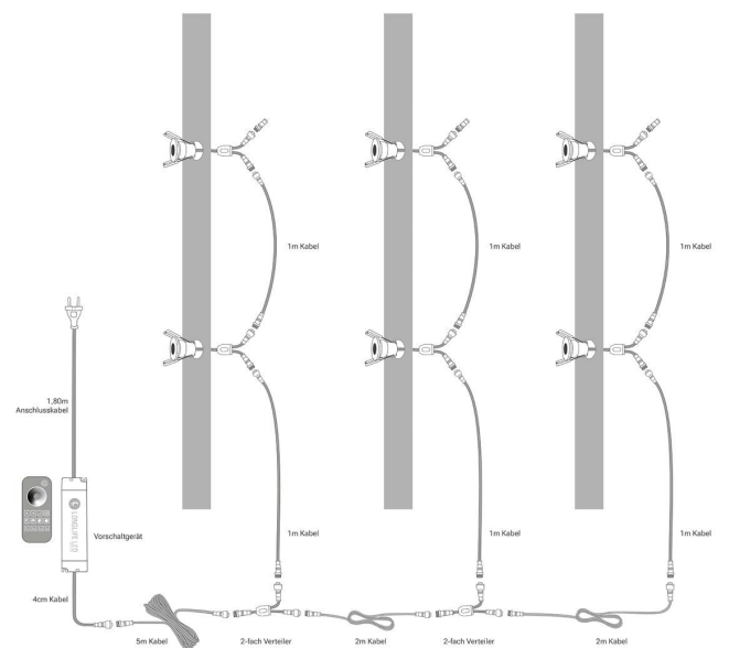
Einbaustrahler 6er Set Installationsbeispiel 2
