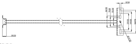
Strahlermontage
