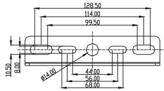
Strahlermontage
